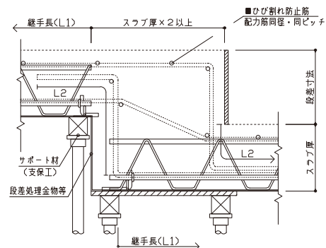
●主筋方向 段差部納まり図 (段差寸法 > 60\text{mm} )
