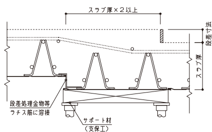
●配力筋方向 段差部納まり図 (段差寸法 \leq 60\text{mm} )
