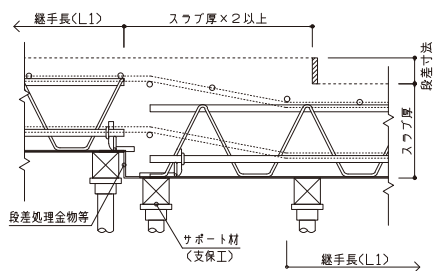
●主筋方向 段差部納まり図 (段差寸法 \leq 60\text{mm} )
