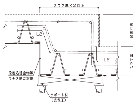
●配力筋方向 段差部納まり図 (段差寸法 > 60\text{mm} )
